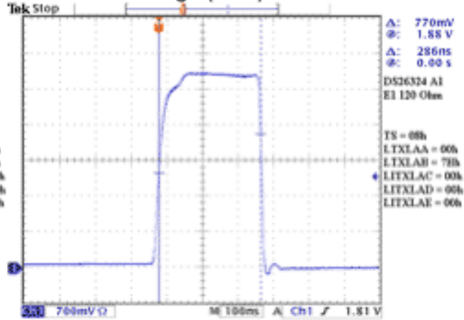
E1 120 Max Plateau (2) Max (2CE)
