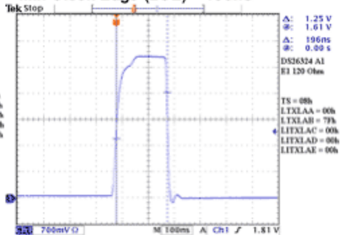
E1 120 Max Plateau (2) Min (2CE)
