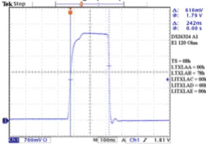
E1 120 Max Plateau (2) Norm (2CE)
