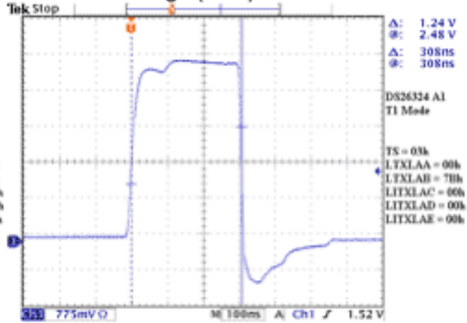
T1 Max Plateau (2) Max (2CE)
