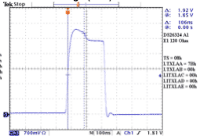
E1 120 Max Overshoot (1) Max (1CE)
