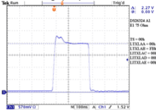
E1 75 Min Plateau (2) Max (2CE)
