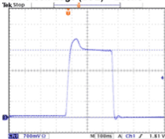
E1 120 Min Plateau (2) Max (2CE)
