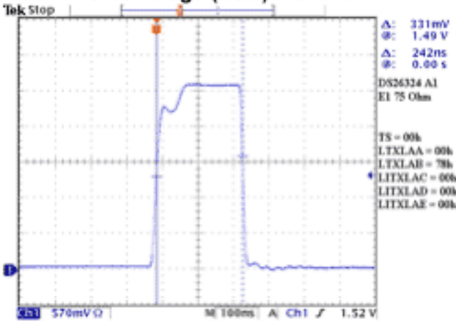
E1 75 Man Plateau (2) Normal (2CE)
