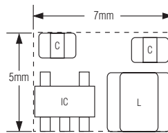
尺寸较大的 SOT23方案 35mm 2
